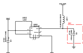
BTP DC-DC
